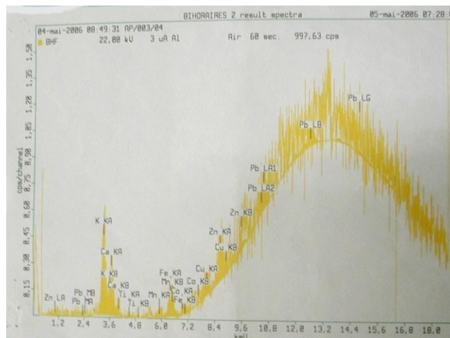
Spectre 3. Identification des éléments minéraux contenus dans l'échantillon EM
