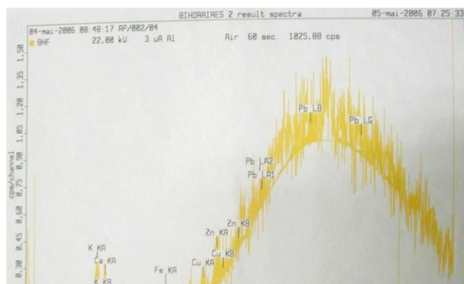
Spectre 1. Identification des éléments minéraux contenus dans l'échantillon Ev
