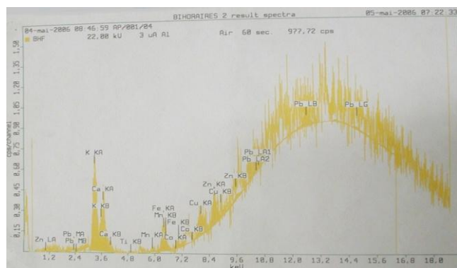
Spectre 1. Identification des éléments minéraux contenus dans l'échantillon Ev
